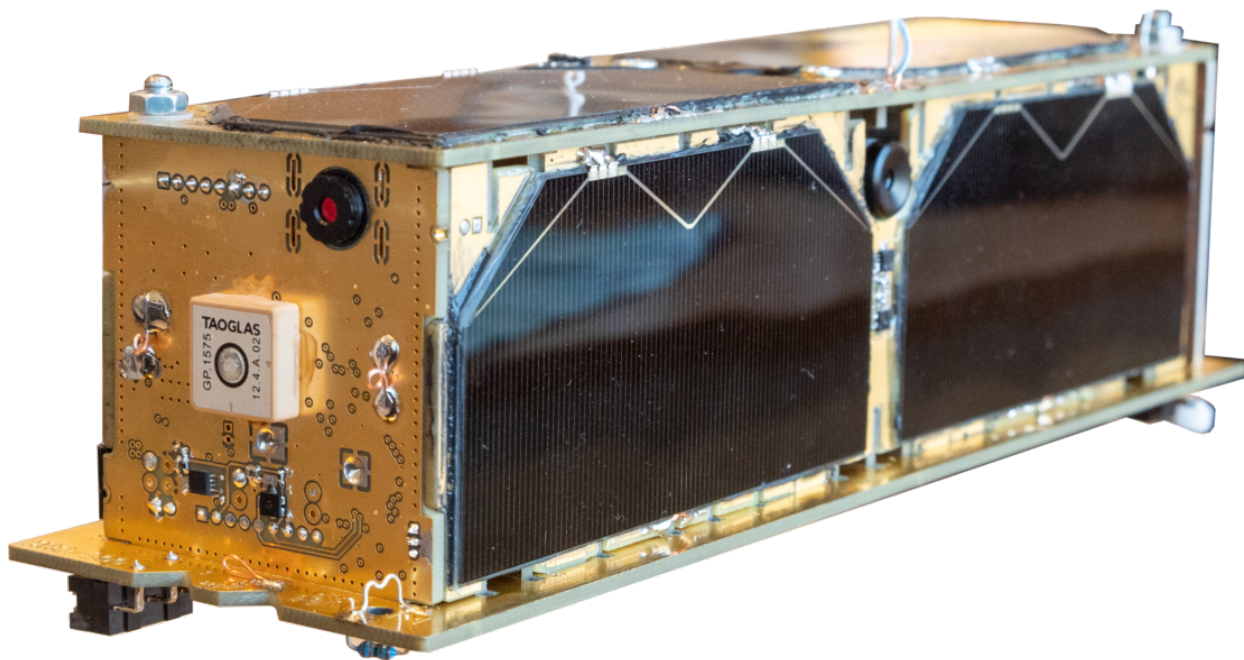
2. ábra. Az MRC-100 összeszerelt állapotban, startra készen - 2022. december
