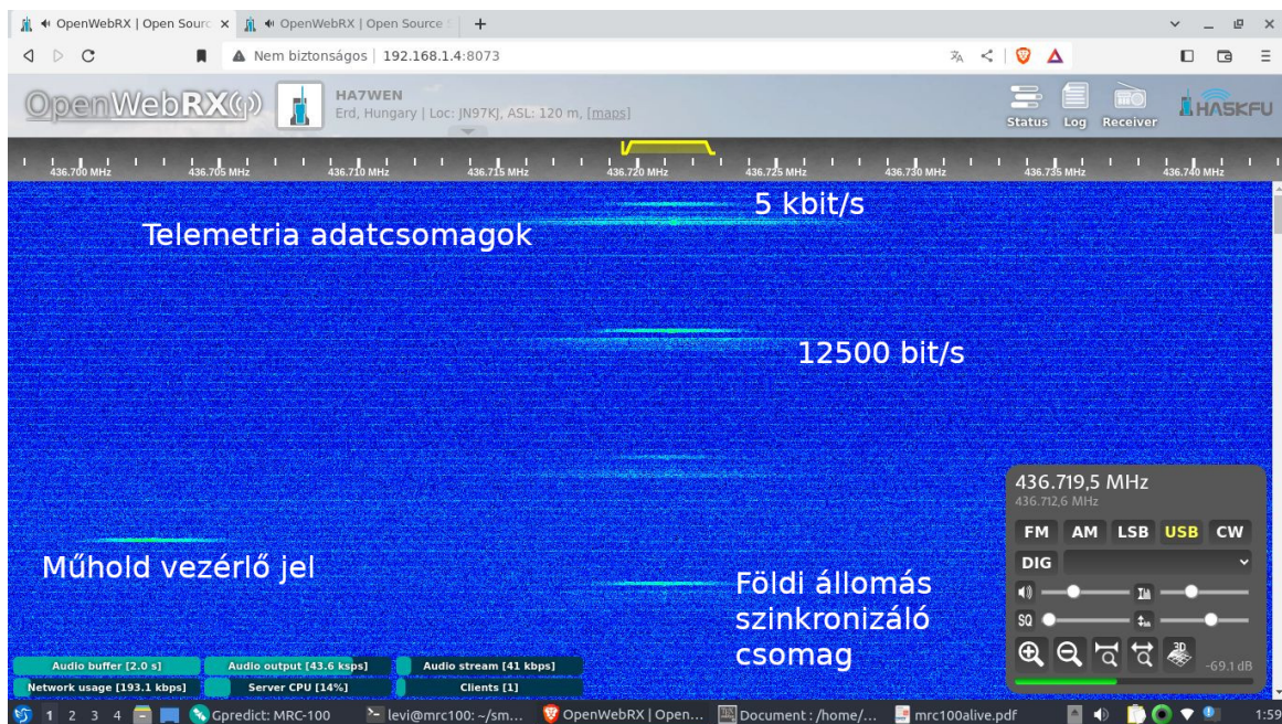
4. ábra. Az MRC-100-ról vett jel vizesés diagramon (frekvencia-idő-amplitúdó)
